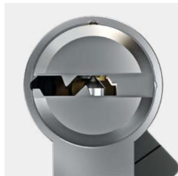
Přední pohled na cylindrickou vložku
