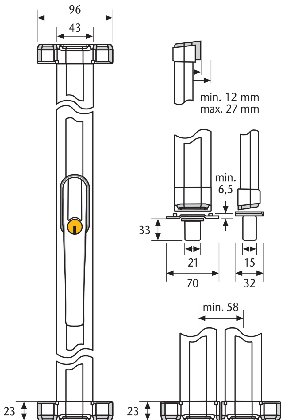
DSB - Uzamykací bod pro dvoukřídlá okna
